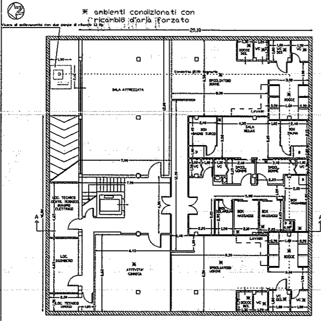
PIANTA SEMINTERRATO SCALA 1:100
